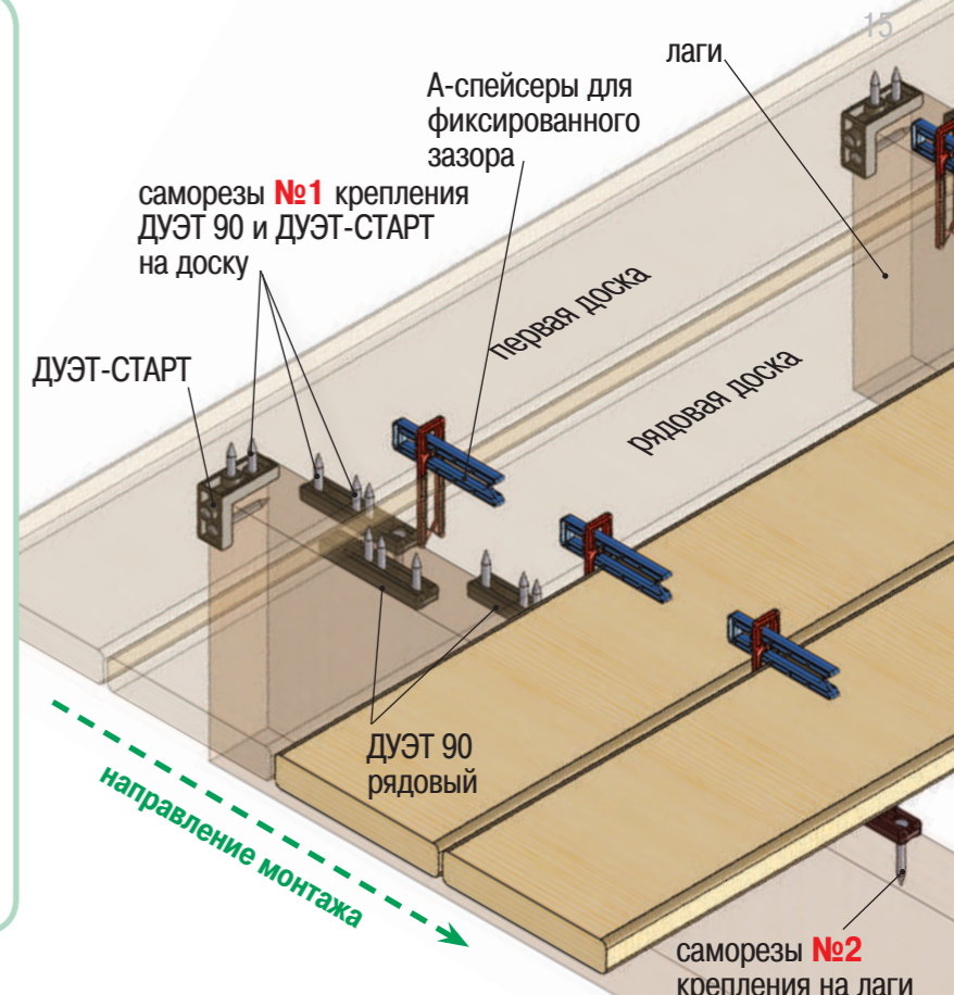
Вариант 2 – БОКОВОЕ крепление стартового крепежа
